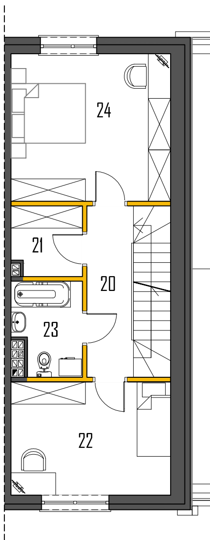
RZUT PODDASZA
