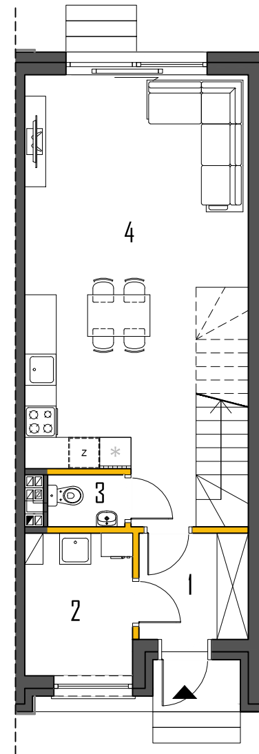
RZUT PARTERU
